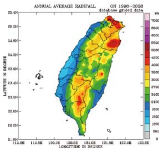
民國85年～97年平均雨量分布圖
