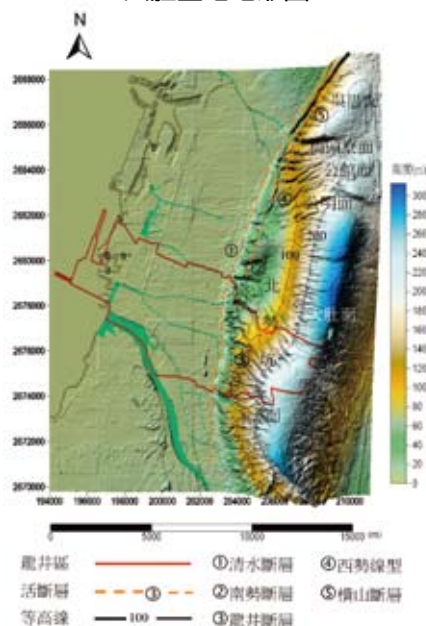
大肚臺地地形圖
